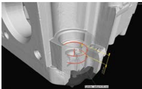
Typická průmyslová aplikace CT - měření vnitřních rozměrů
